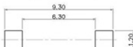
P.C.B LAND PATTERN
